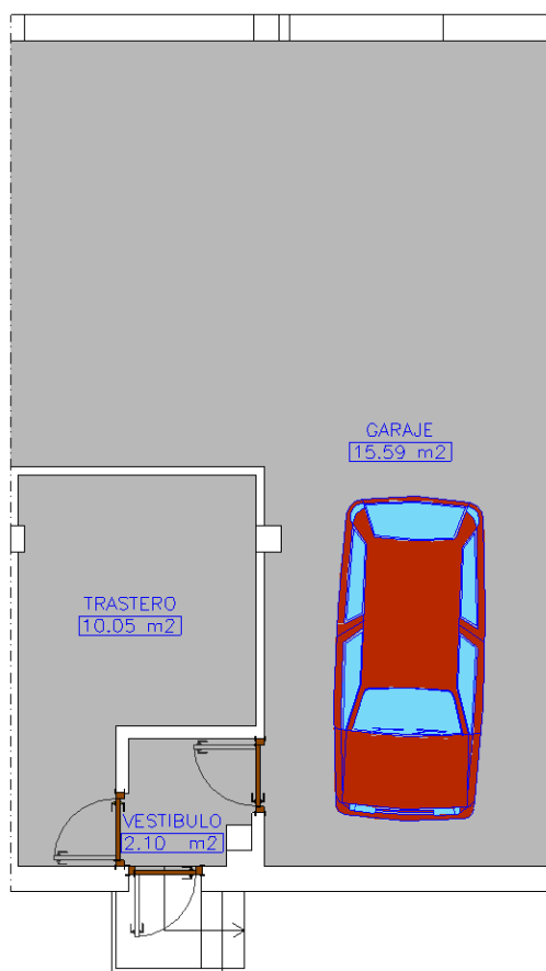
PLANTA GARAJE
